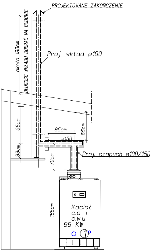
SZCZEGÓŁY KOMINA DOBRAĆ NA BUDOWIE
